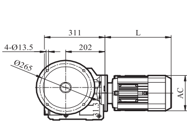
GKA77T
