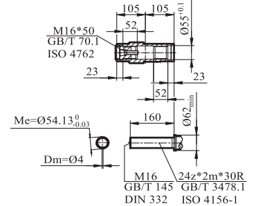
GKV/GKVZ/GKV77输出轴
