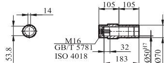
GKA/GKAZ/GKAF77输出轴
