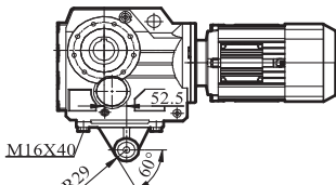
GKA/GKAZ/GKAF77输出轴
