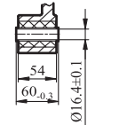
GKV/GKVZ/GKV77输出轴
