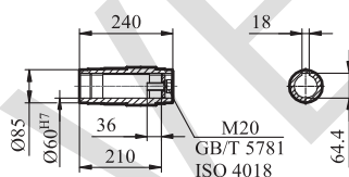
GFA/GFAZ/GFAF87输出轴
