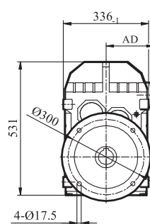
GFV/GFVZ/GFVF87输出轴
