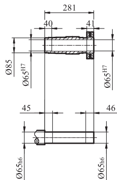
GFH/GFHZ/GFHF87输出轴
