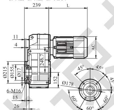
GFAZ/GFHZ/GFVZ87
