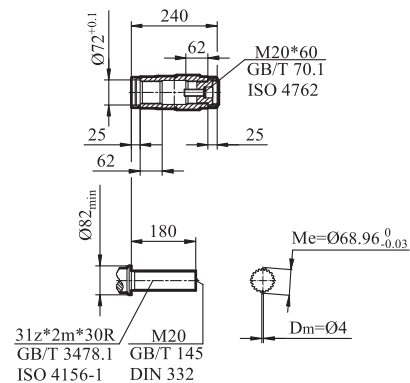
GFV/GFVZ/GFVF87输出轴
